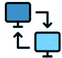
Réseaux informatiques
